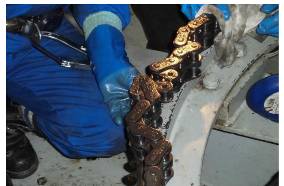
(原動滑車駆動チェーン交換作業)
