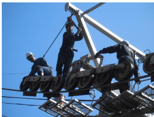
(支柱索輪交換作業)
